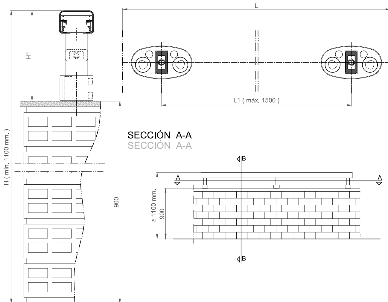
SECCIÓN B-B SECTION B-B
